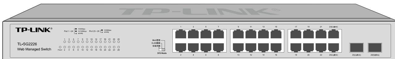
图 2-1 TL-SG2226前面板
