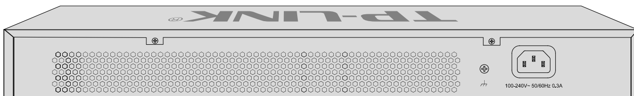
图 2-7 TL-SG2226后面板
