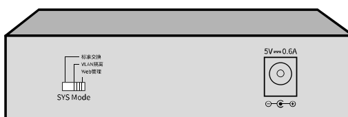
图 2-9 TL-SG2005后面板
